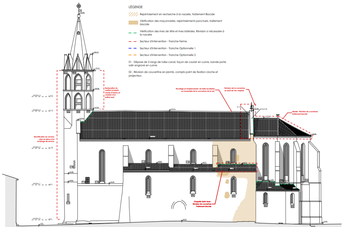
Élévation sud
