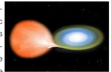
Super Nova de type I
